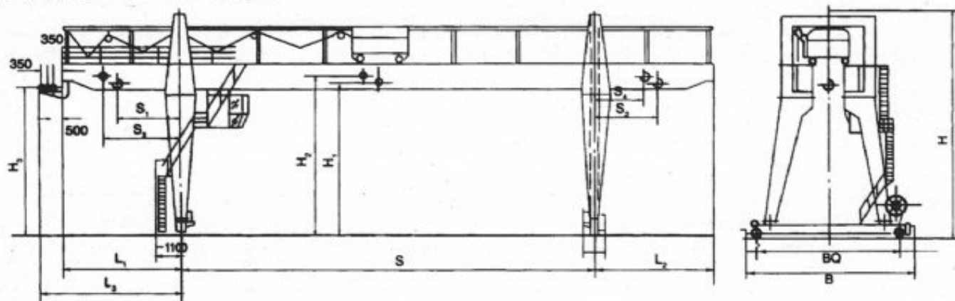
外形尺寸图: Outer size Diagram
